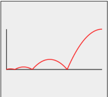
Bounce.easeIn
