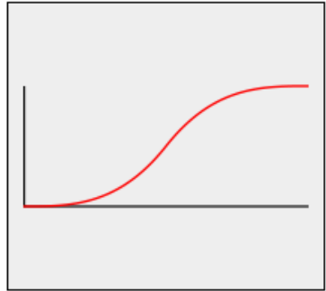
Cubic.easeInOut
