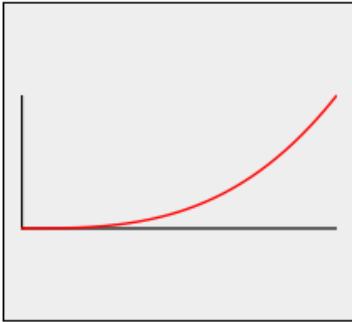
Cubic.easeIn
