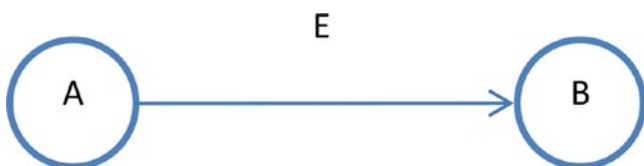
Figure 9-7. An EdgeTriplet
