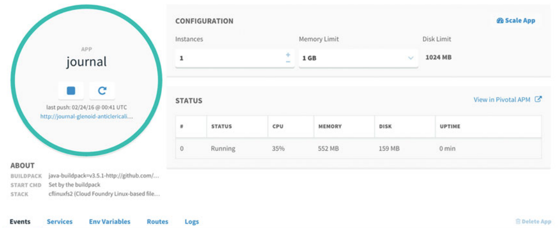
Figure 13-9. Journal App
